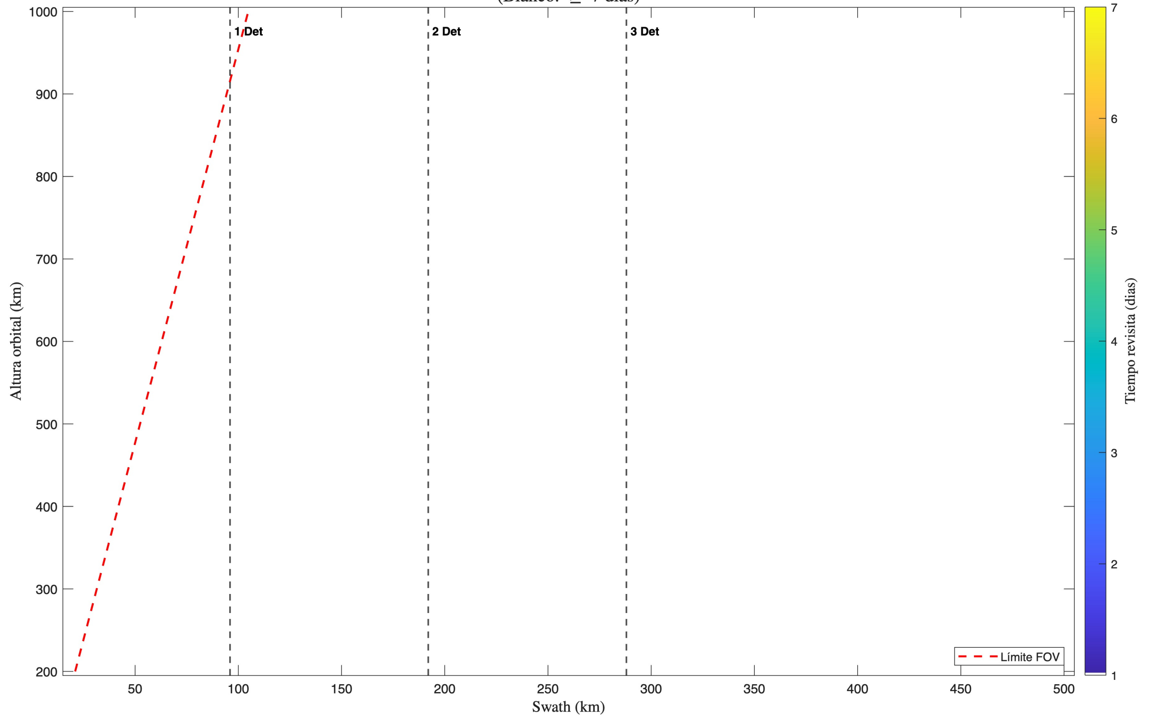
Tiempo Revisita - 1 Satelite(s); 2 Telescopio(s): Cassegrain; Detector 1 (Blanco: \geq 7 dias)
